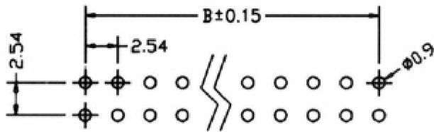
P.C.Board Layout
