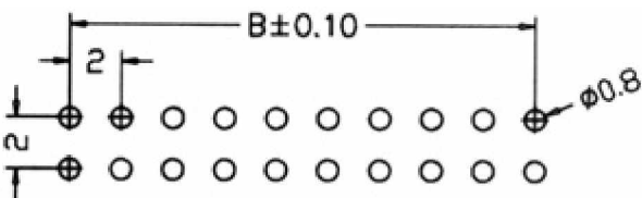
P.C.Board Layout
