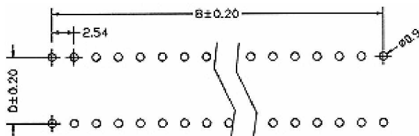
P.C.Board Layout
