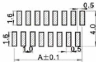
正针 PCB 寸法 Positive needle PCB LAYOUT
