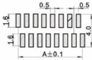
反针 PCB 寸法 Versa needle PCB LAYOUT
