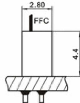
安装图 ASSEMBLY LAYOUT
