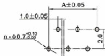
正针 PCB 寸法 Positive needle PCB LAYOUT
