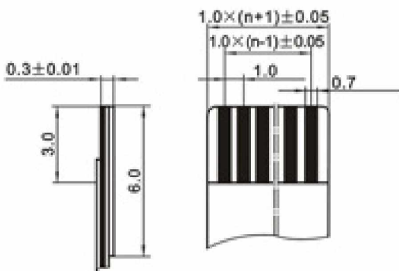
适用扁平电缆 Proper cable
