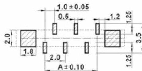
正针 PCB 寸法 Positive needle PCB LAYOUT
