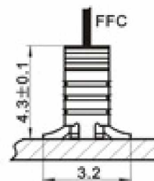
安装图 ASSEMBLY LAYOUT
