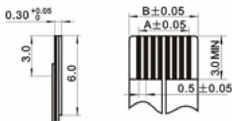
适用扁平电缆 Proper cable
