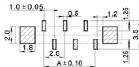
反针 PCB 寸法 Versa needle PCB LAYOUT
